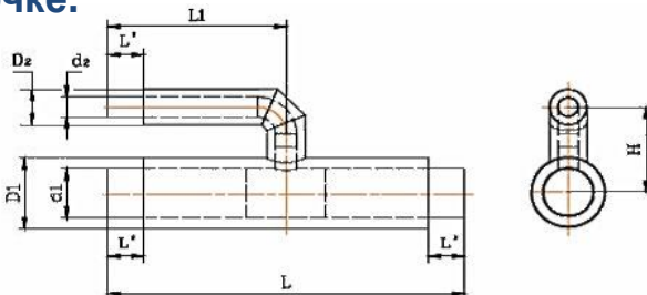
d2,mm d1,mm 32 38 45 57 76 89 108 133 159 219 273 325 426 530 630 720 820 920 1020 1220 1420 L 1200 1200 1200 1200 1300 1300 1300 1400 1400 1800 1800 1900 2000 2000 2000 2000 2100 2100 2400 2700 32 L2 H 700 275 700 275 700 275 700 283 700 293 700 303 700 313 700 325 700 338 700 370 700 413 700 438 700 493 - - - - - - - - 38 L2 H - 700 275 700 275 700 283 700 293 700 303 700 313 700 325 700 338 700 370 700 413 700 438 700 493 - - - - - - - - 45 L2 H - - 700 275 700 283 700 293 700 303 700 313 700 325 700 338 700 370 700 413 700 438 700 493 - - - - - - - - 57 L2 H - - - 700 290 700 300 700 310 700 320 700 333 700 345 700 378 700 420 700 445 700 500 - - - - - - - - 76 L2 H - - - - 700 310 700 320 700 330 700 343 700 355 700 388 700 430 700 455 700 510 700 585 - - - - - - - 89 L2 H - - - - - 700 330 700 340 700 353 700 365 700 398 700 440 700 465 700 520 700 595 700 640 - - - - - - 108 L2 H - - - - - - 700 350 700 363 700 375 700 408 700 450 700 475 700 530 700 605 700 650 700 700 - - - - - 133 L2 H - - - - - - - 800 375 800 388 800 420 800 463 800 488 800 543 800 618 800 663 800 713 800 763 - - - - 159 L2 H - - - - - - - - 800 405 800 435 800 475 800 500 800 555 800 630 800 675 800 725 800 775 800 825 - - - 219 L2 H - - - - - - - - - 800 565 800 608 800 633 800 688 800 763 800 808 800 858 800 908 800 958 800 1008 - - 273 L2 H - - - - - - - - - - 1000 650 1000 675 1000 730 1000 805 1000 850 1000 900 1000 950 1000 1000 1000 1050 1000 1100 1000 1150 325 L2 H - - - - - - - - - - - 1100 713 1100 763 1100 830 1100 875 1100 925 1100 975 1100 1025 1100 1075 1100 1125 1100 1175 426 L2 H - - - - - - - - - - - - 1200 913 1200 985 1200 1030 1200 1080 1200 1130 1200 1180 1200 1230 1200 1330 1200 1430 530 L2 H - - - - - - - - - - - - - 1200 1160 1200 1205 1200 1255 1200 1305 1200 1355 1200 1405 1200 1505 1200 1605 630 L2 H - - - - - - - - - - - - - - 1200 1250 1200 1300 1200 1350 1200 1400 1200 1450 1200 1550 1200 1650 720 L2 H - - - - - - - - - - - - - - - 1200 1500 1200 1550 1200 1600 1200 1650 1200 1850 1200 1950 820 L2 H - - - - - - - - - - - - - - - - 1200 1800 1200 1850 1200 1900 1200 2000 1200 2100 920 L2 H - - - - - - - - - - - - - - - - - 1300 2000 1300 2050 1300 2150 1300 2250 1020 L2 H <
